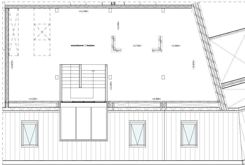
Plattegrond verdieping 04 1:50
