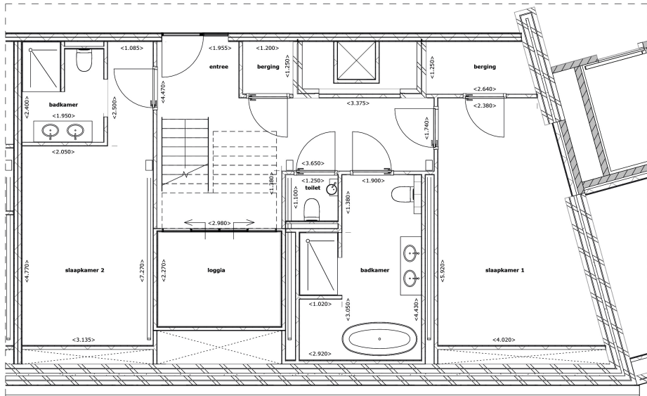
Plattegrond verdieping 03 1:50
